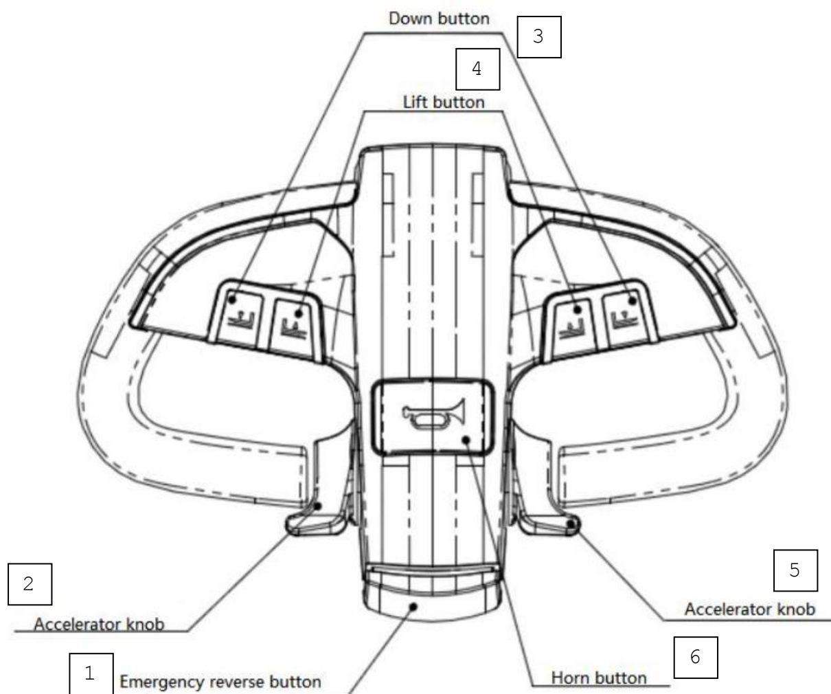
Рис. Рукоятка управления:
