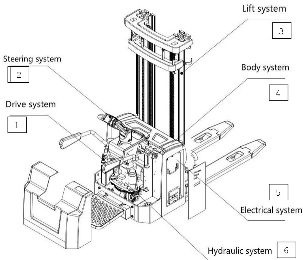
Рис. Штабелер в сборе:
