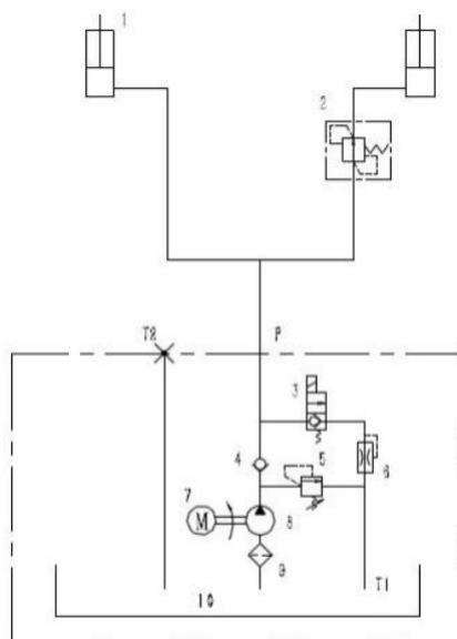
Рис. Серия MBF01. Схема
